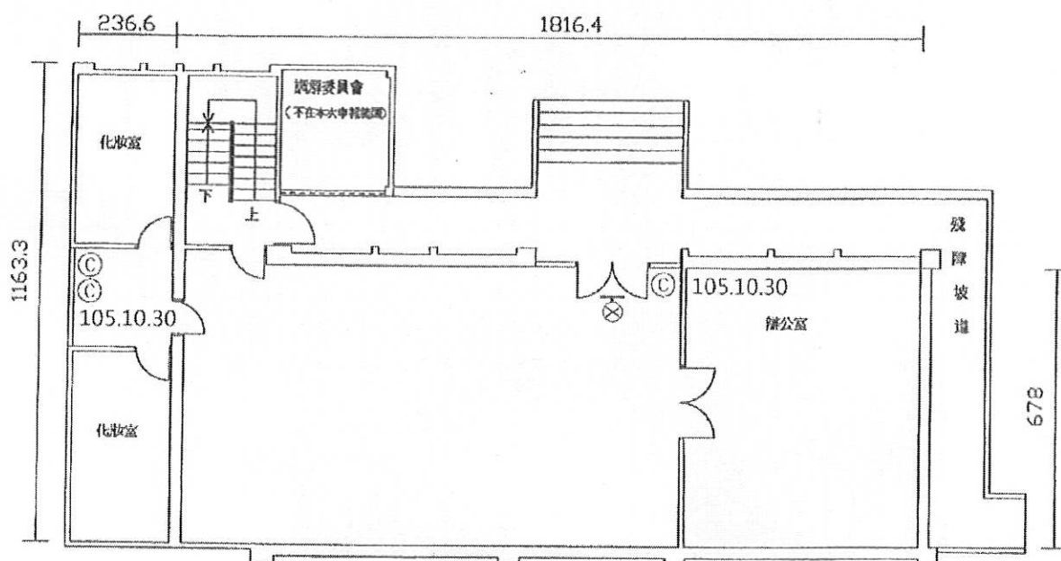
一樓平面圖 註1：本次以雷射丈量尺寸，電腦計算面積(不含牆厚，調解委員會及安全梯面積)，面積：148.66m 2 。
